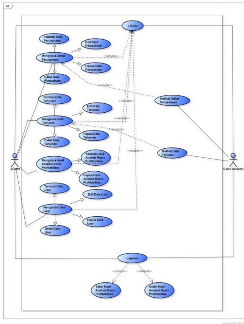
Gambar 1. Rancangan Usecase Diagram
