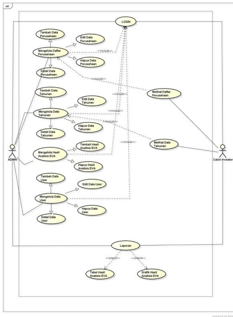
Gambar 1. Rancangan Usecase Diagram
